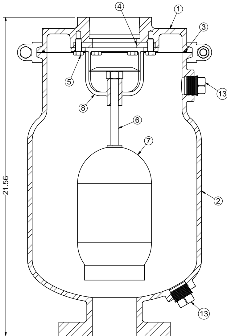
SECTION A-A
