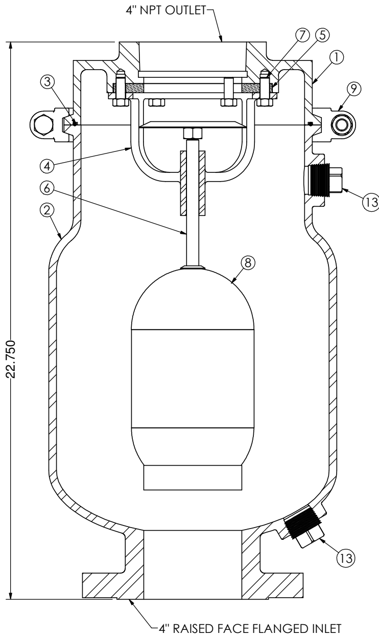
SECTION A-A
