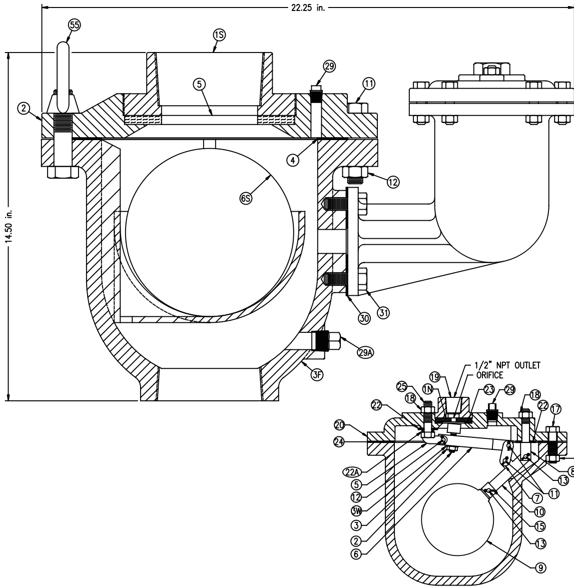
SECTION A-A
