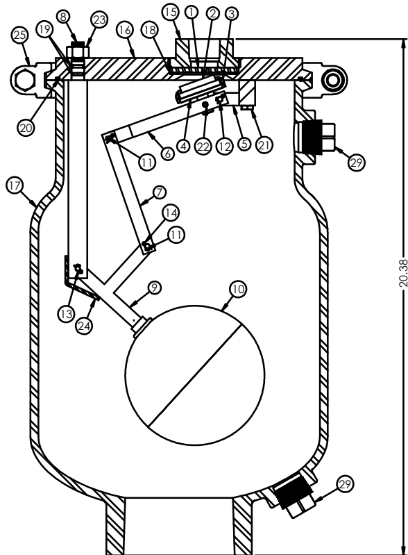
SECTION A-A
