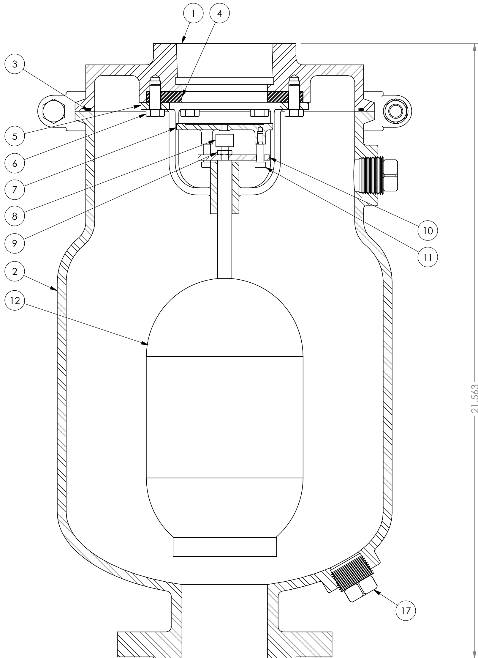
SECTION A-A
